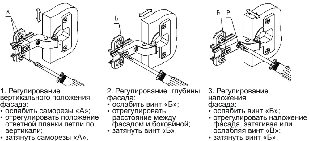
Схема 3. Регулирование зазоров и положения фасада
