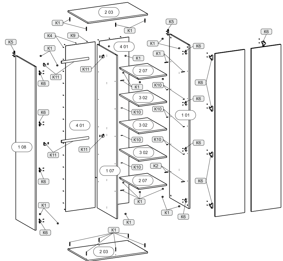
Общий вид Схема 1. Сборка шкафа (левая)
