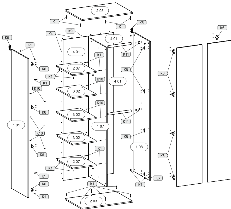
Общий вид Схема 1. Сборка шкафа (правая)
